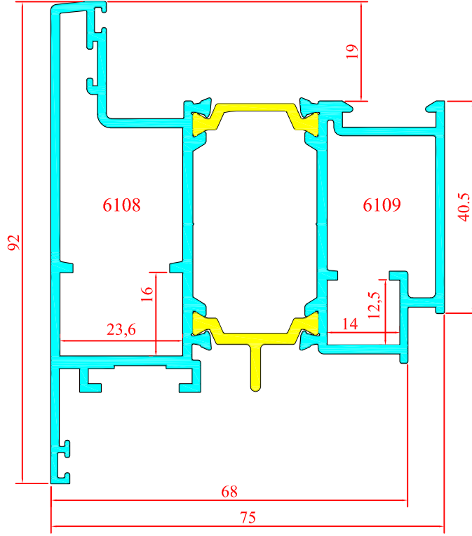
YAS 68 - 05 DIŞA AÇILIM KAPI KANAT PROF. 2.110 Kg/m
