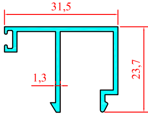
AS 01 6251 ÇİFT CAM ÇITA PROF. 0.317 Kg/m
