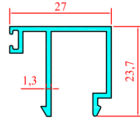
AS 01 6253 ÇİFT CAM ÇITA PROF. 0.300 Kg/m
